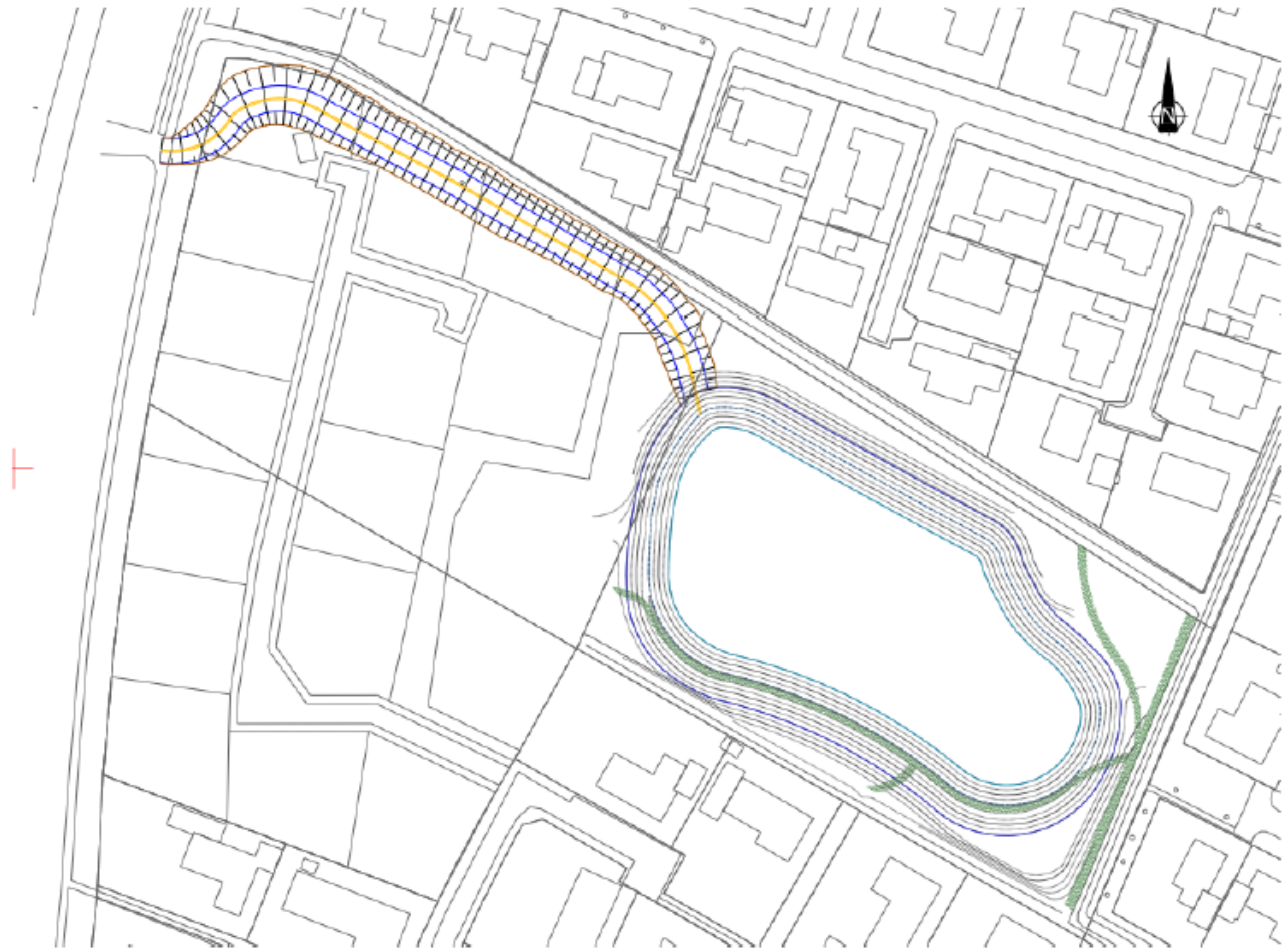
Figur 1.2: Udformning af bassin.
