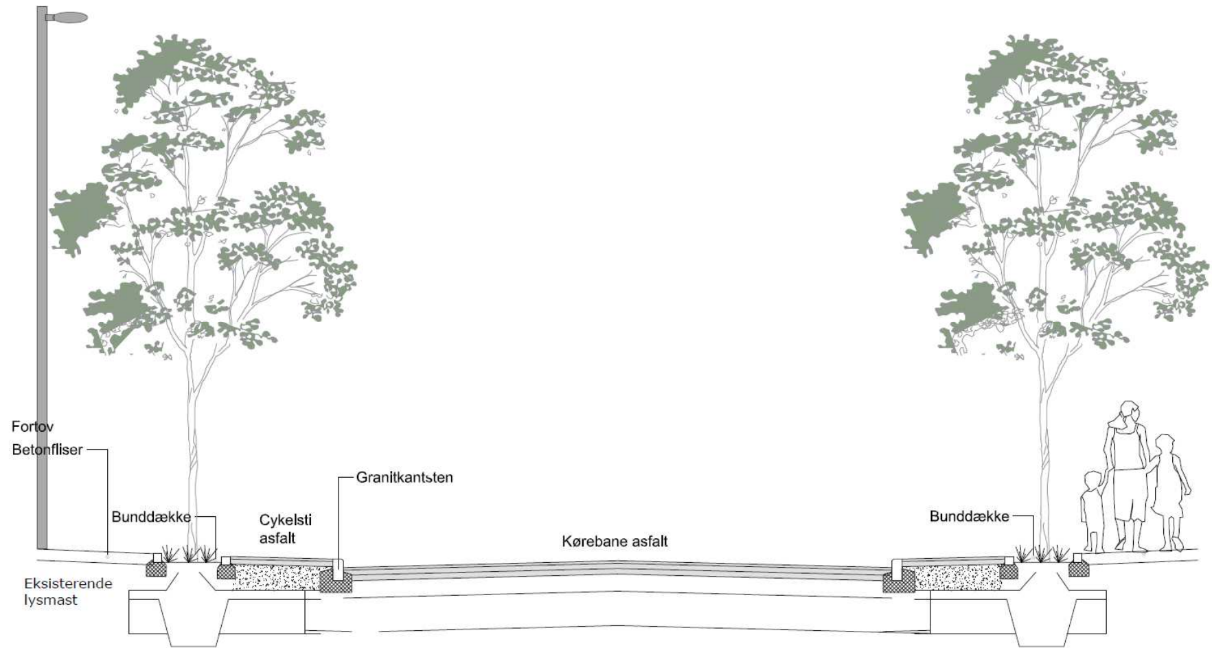
Tværsnit Tjørring Hovedgade Juni, 2016
